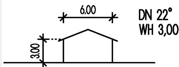
SCHEMASCHNITT GARAGE
