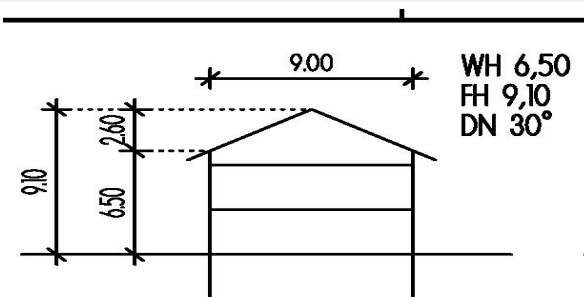
SCHEMASCHNITT EINFAMILIENHAUS
