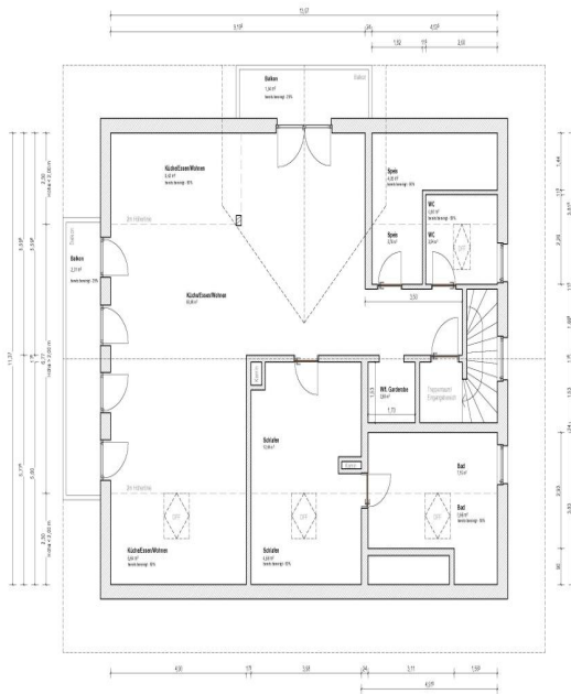
Grandes Dachgeschoss M 1:100
